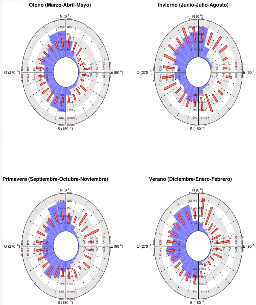
Figura 10: Rosa de la velocidad de viento a 93 metros. Las barras azules indican el porcentaje de los valores horarios según la dirección del viento. Las barras rojas indican el rango inter-cuartil de velocidad de viento para cada intervalo de dirección. La dirección de viento es un ángulo que indica el sector desde donde proviene el viento. En particular: para 0 el viento viene del Norte; para 90 se tiene viento del Este; en el caso de 180 el viento es del Sur; y para 270 se tiene viento del Oeste.
